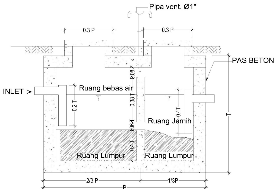
POTONGAN A-A
