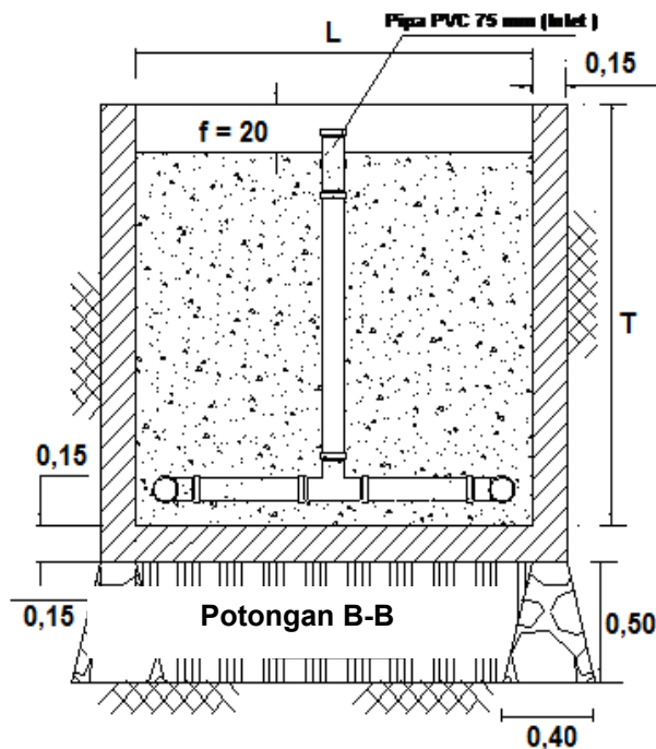
Gambar 8 – Kolam sanita (lanjutan)
