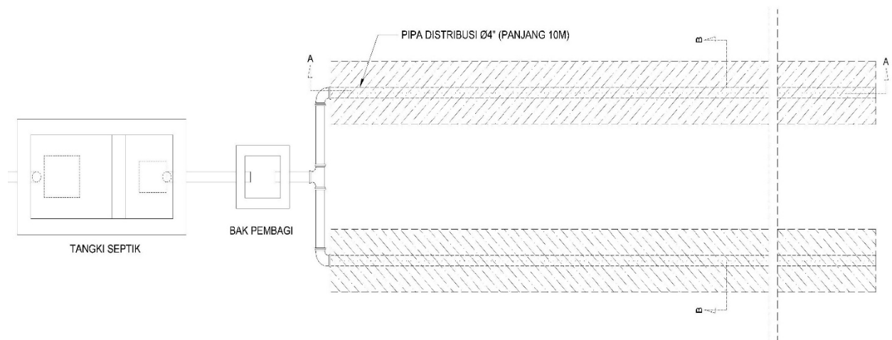
DENAH TANGKI SEPTIK DENGAN BIDANG RESAPAN
