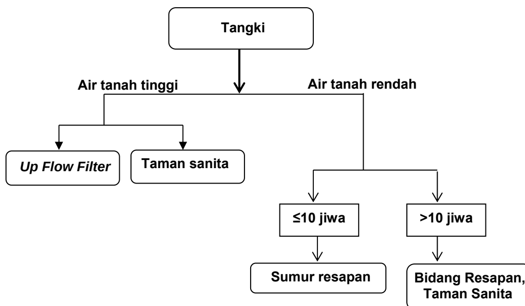
Gambar 1 – Alternatif pengolahan lanjutan efluen tangki septik
