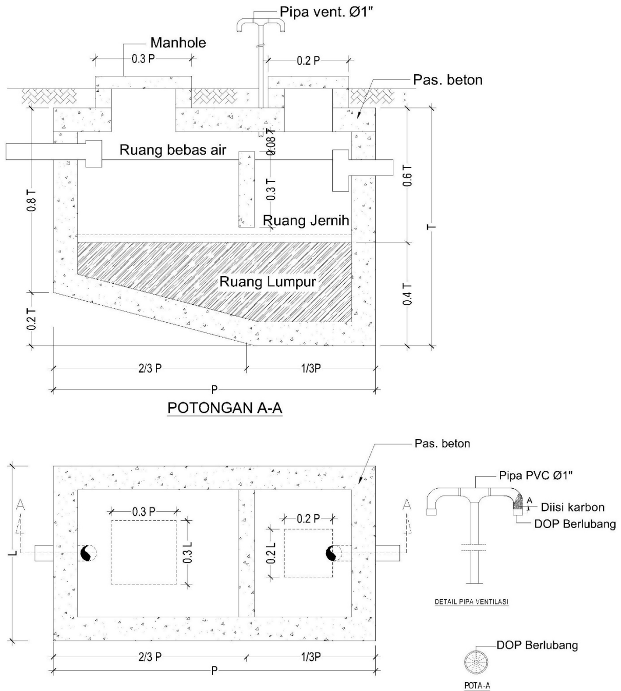
DENAH TANGKI SEPTIK SATU KOMPARTEMEN
